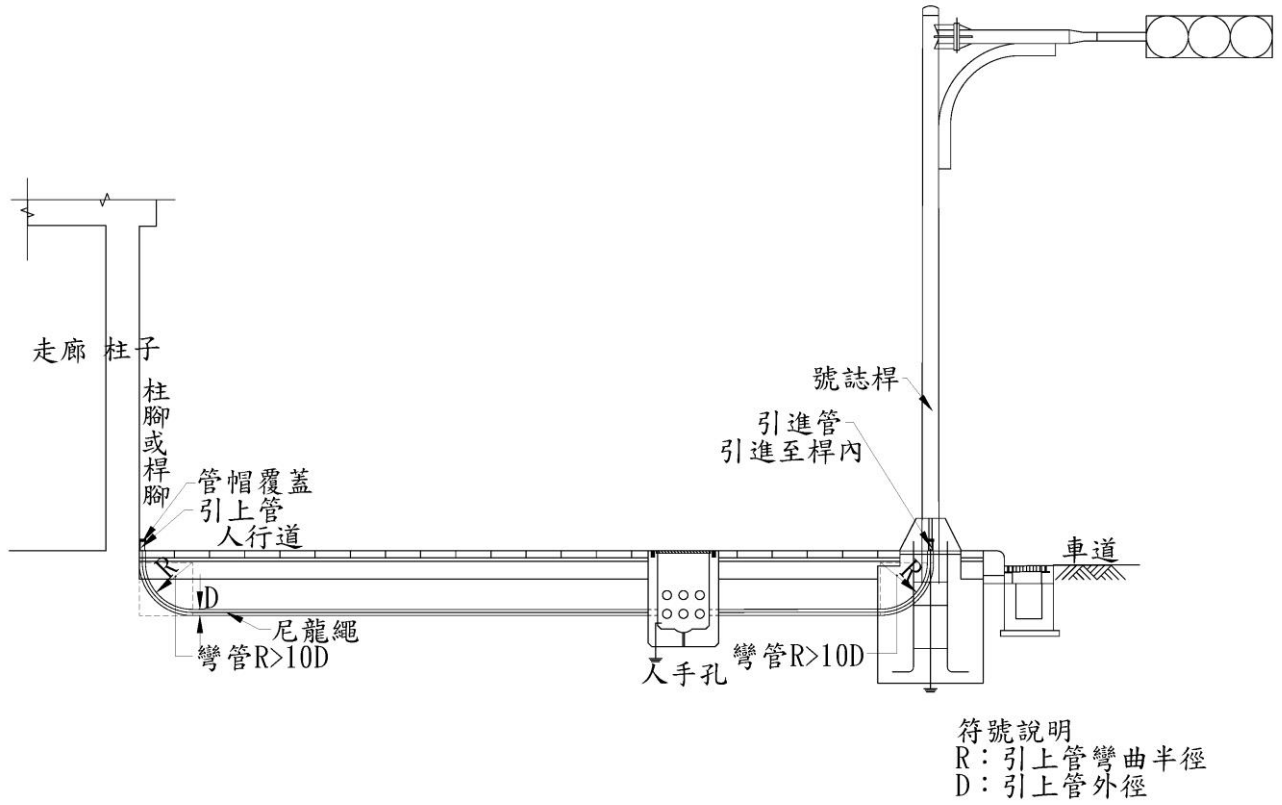
圖 21.3.2 引上管、引進管配置參考圖
